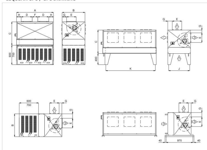
ESQUEMA GPC / GPC DRAWING
