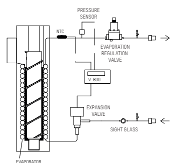
GIQ CO 2 REFRIGERATION CIRCUIT CIRCUITO REFRIGERACIÓN GIQ CO 2 CIRCUIT RÉFRIGÉRANT GIQ CO 2 KÜHLKREISLAUF GIQ CO 2
