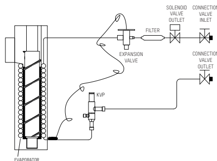
GIQ R404 REFRIGERATION CIRCUIT CIRCUITO REFRIGERACIÓN GIQ R404A CIRCUIT RÉFRIGÉRANT GIQ R404A KÜHLKREISLAUF GIQ R404A
